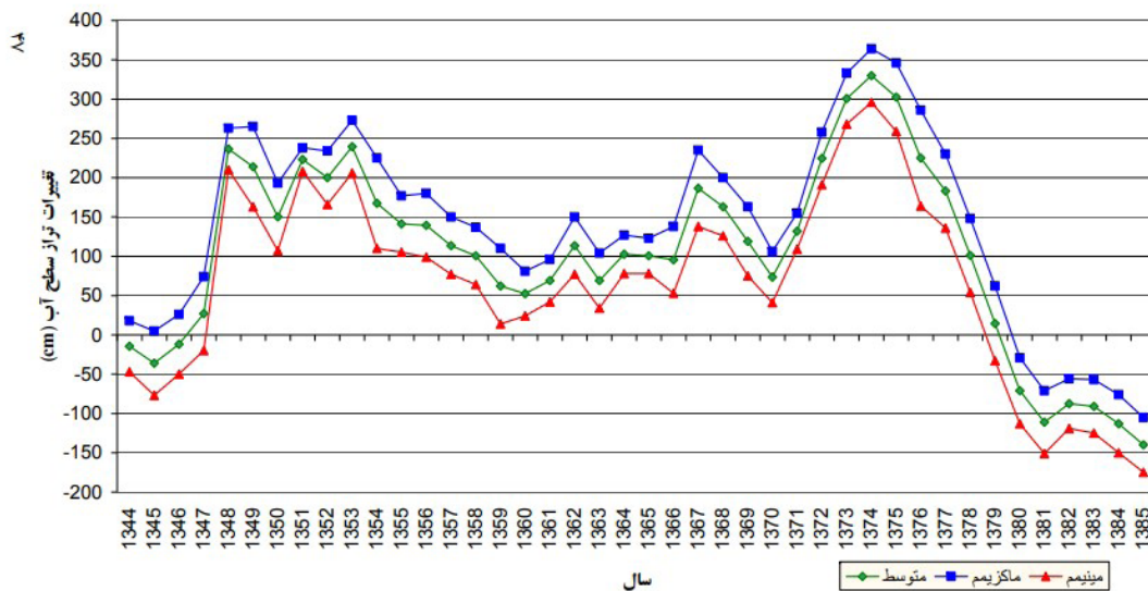
نمودار شماره (۴-۲) - تغییرات تراز سطح آب دریاچه ارومیه بر مبنای اشل معاونت مطالعات شرکت آب منطقه‌ای آذربایجان غربی
